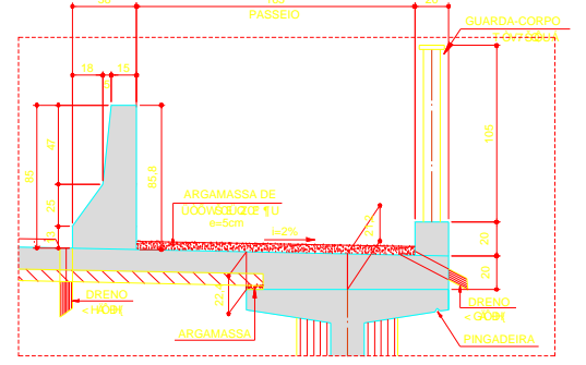
ΔΕΤΑΛΗ 04 ESC. 1:25
