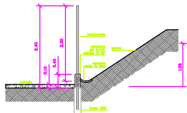
CORTE DO ALAMBRADO NO LOCAL COM TALUDE ESC.: 1:50
