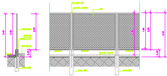
CORTE DO ALAMBRADO ESC.: 1:50
