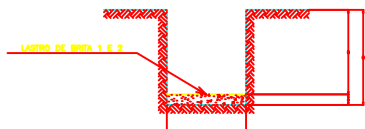
CORTE ESQUEMÁTICO DE VALA ESC. 1:50
