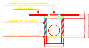
POÇO DE VISITA-CORTE ESC. 1:50
