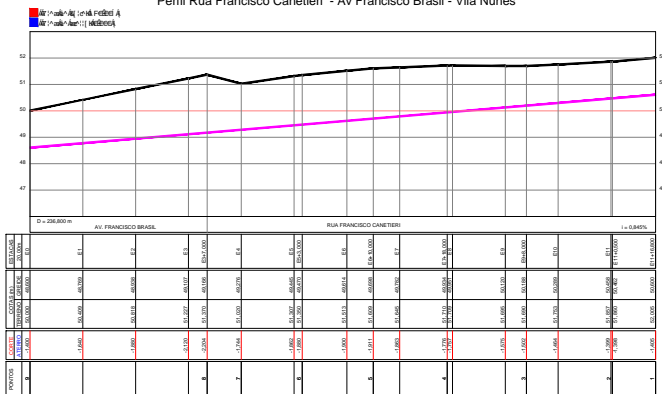
Perfil Rua Francisco Canetieri - Av Francisco Brasil - Vila Nunes
